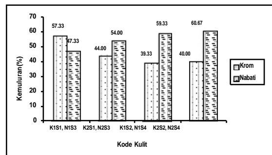
Gambar 2 : Kemuluran ( % )
